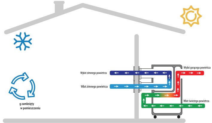
KLIMATYZATOR NA ZEWNĄTRZ POMIESZCZENIA OPCJA Z ADAPTEREM PLENUM OBIEGU ZIMNEGO POWIETRZA WZROST EFEKTYWNOŚCI O 60% ZNACZNIE CICHSZA PRACA
